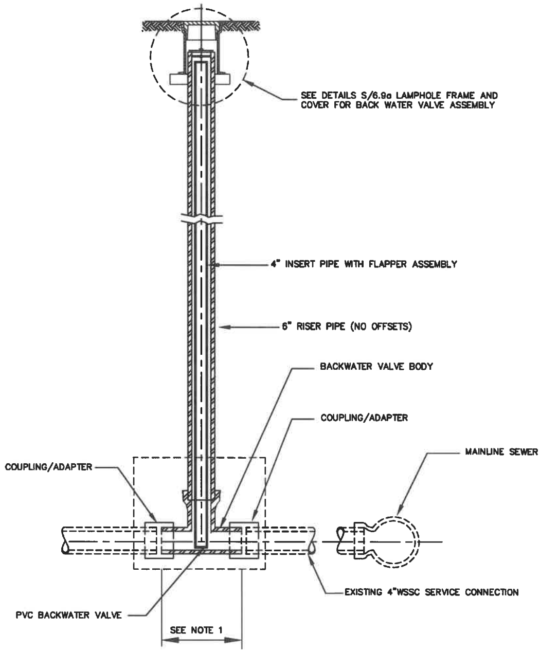
ELEVATION
